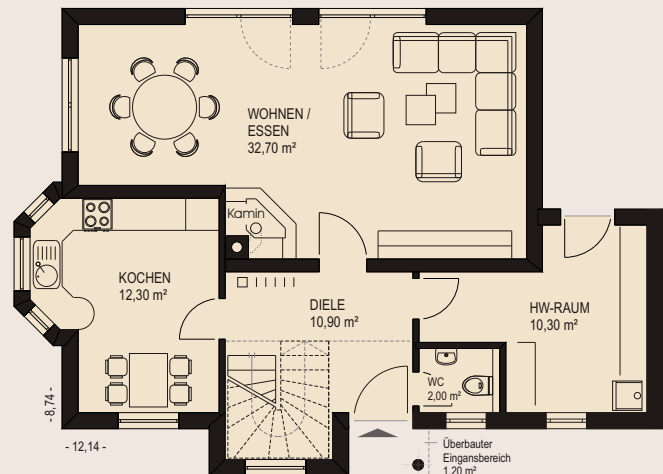
ERDGESCHOSS FLÄCHE : 69,40 m 2
